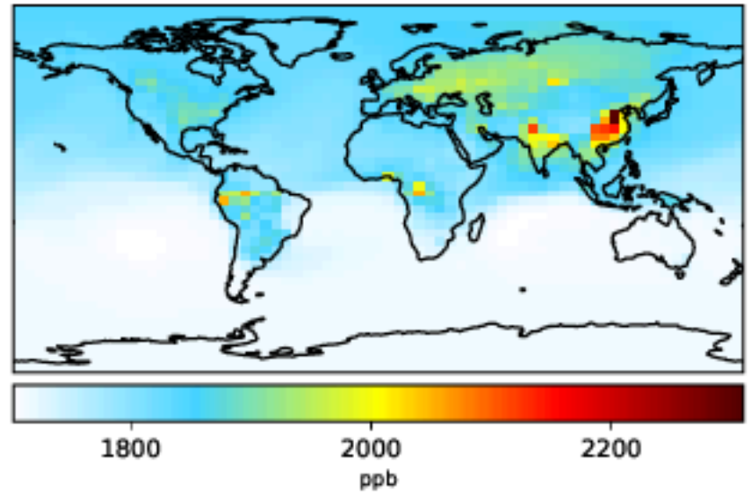
gcc_CH4 (Dev) 4.0x5.0
