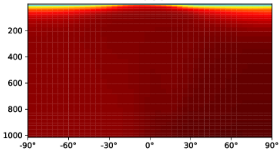
gcc_carbon_CH4 (Ref) 4.0x5.0
