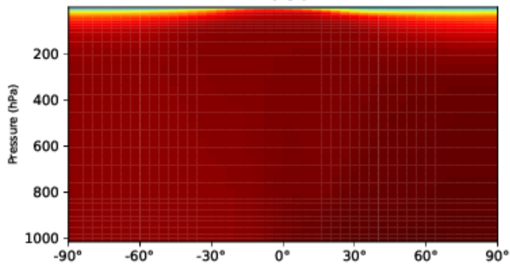
gcc_CH4 (Dev) 4.0x5.0
