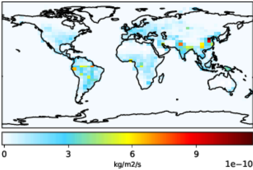
gcc_carbon_CH4 (Ref) 4.0x5.0
