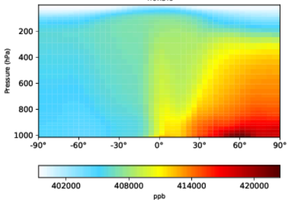
gcc_CO2 (Dev) 4.0x5.0
