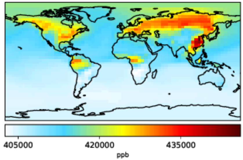
gcc_CO2 (Dev) 4.0x5.0
