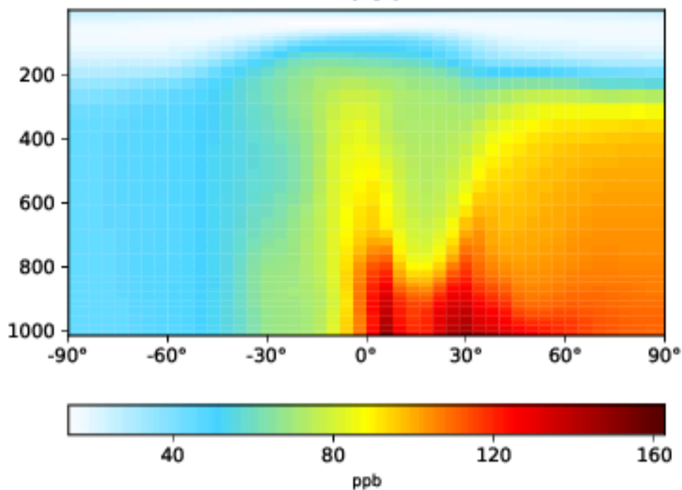
gcc_carbon_CO (Ref) 4.0x5.0
