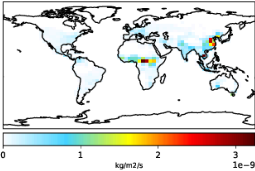
gcc_carbon_CO (Ref) 4.0x5.0
